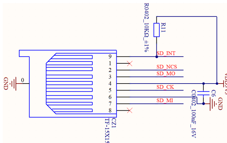
图 3-3 SD 卡座电路示意
