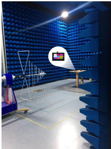
图 6-4 RE 测试图
