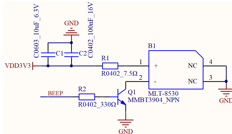
图 3-2 蜂鸣器电路示意
