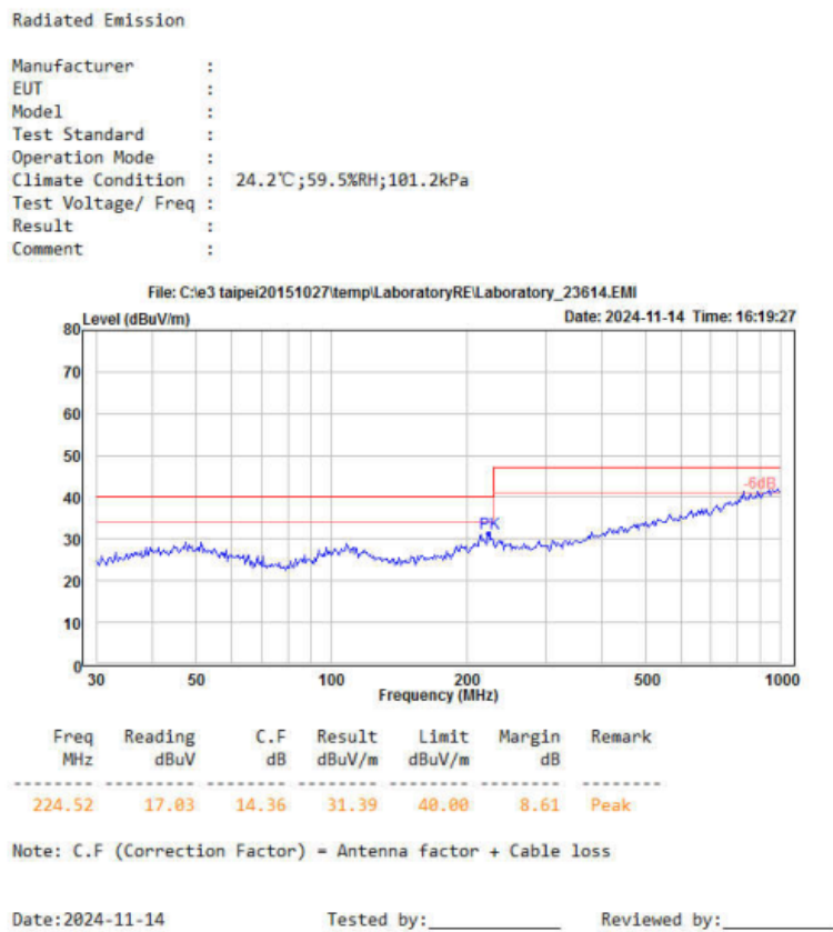
图 6-5 RE 测试水平方向
