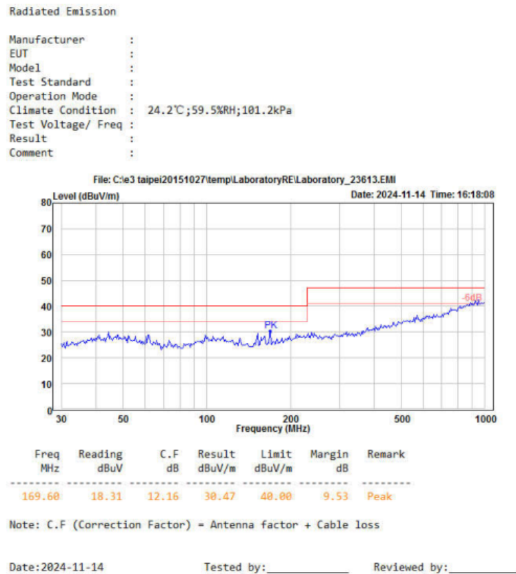
图 6-6 RE 测试垂直方向
